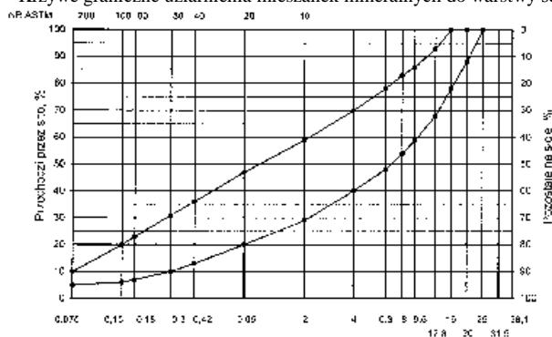
rys. 1. Krzywe graniczne uziarnienia mieszanki mineralnej BA od 0 do 20 mm do warstwy ścieralnej nawierzchni drogi o obciążeniu ruchem dla KR1 i KR2
