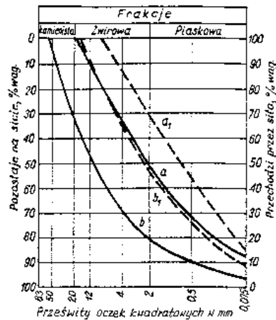
Rysunek 1. Obszar uziarnienia optymalnych mieszanek żwirowych
