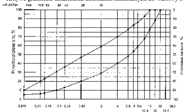
ys. 1. Krzywe graniczne uziarnienia mieszanki mineralnej BA od 0 do 20 mm do warstwy ścieralnej nawierzchni drogi o obciążeniu ruchem dla KR1 i KR2
