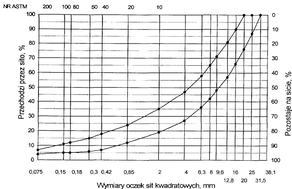
Rys. 1. Krzywe graniczne uziarnienia mieszanki mineralnej BA od 0 do 25 mm podbudowy nawierzchni drogi o obciążeniu ruchem od KR 3
